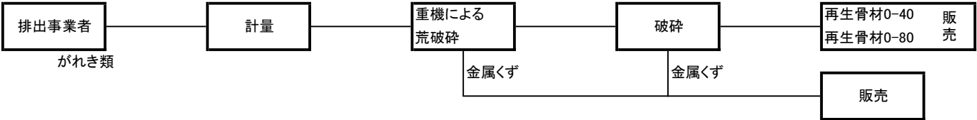
ガラスくず・コンクリートくず及び陶磁器くず、がれき類の破碎施設(札幌)
