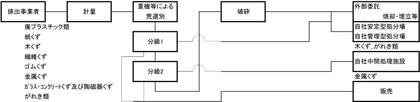
分級選別施設(札幌)
