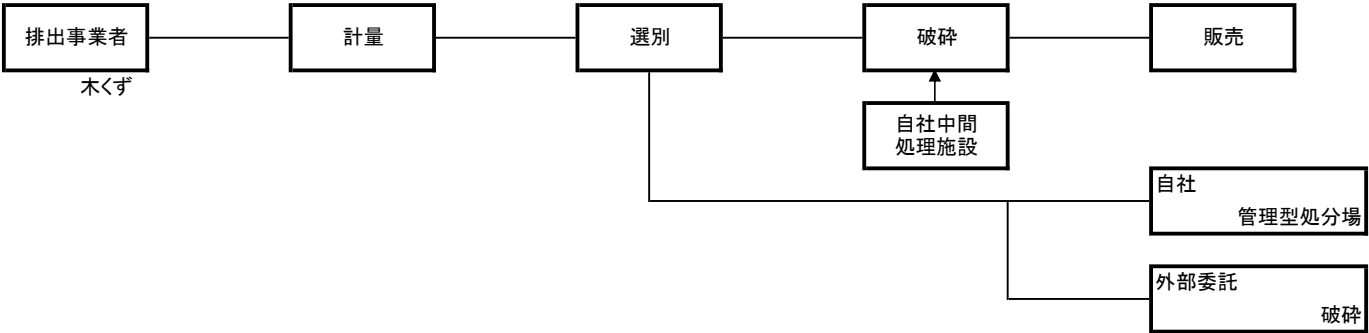
分級選別・破碎施設(登別)
